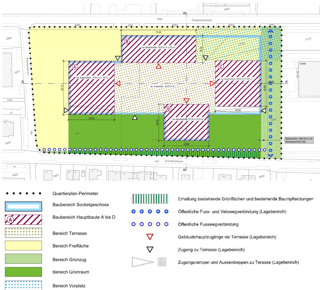
Abbildung 6 Situation Quartierplan (Quelle: Stierli + Ruggli Ingenieure + Raumplaner AG, 20. November 2019)
