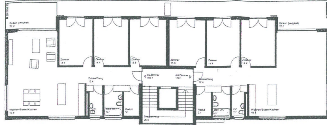
1.+2. OBERGESCHOSS
